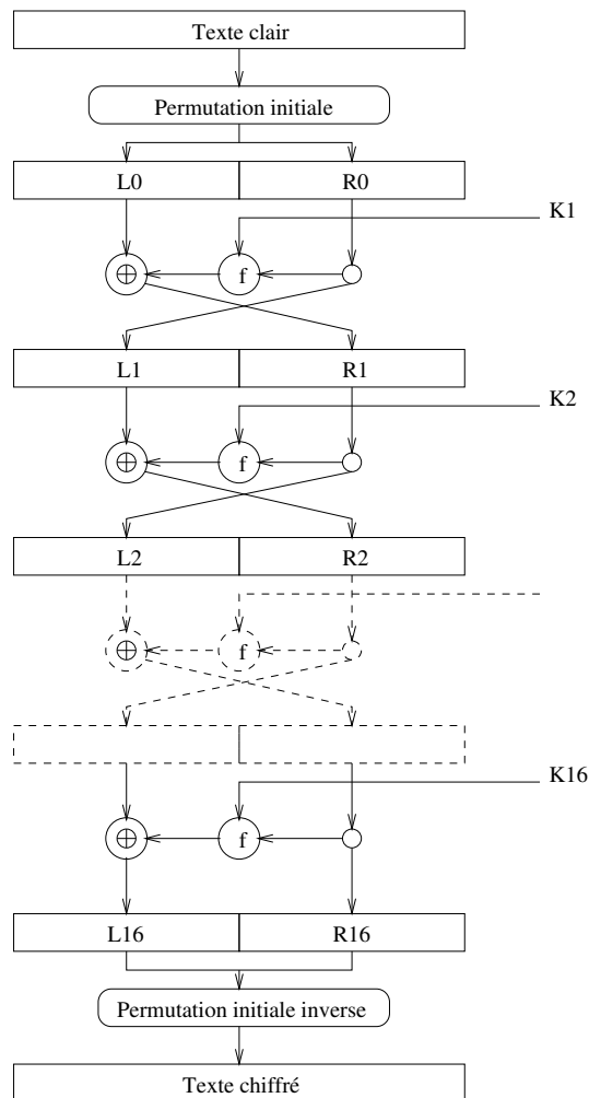
Figure 1. DES : Schéma général
