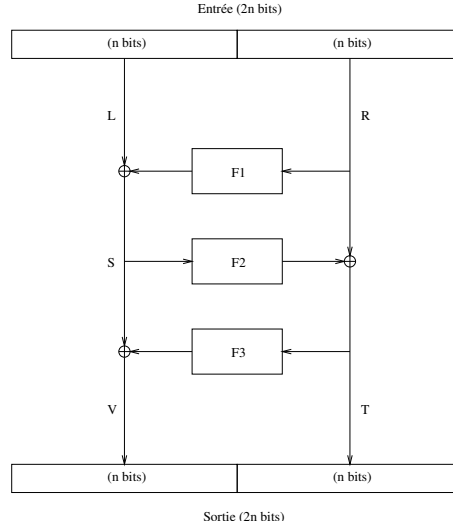
Figure 12. Construction de Luby & Rackoff : \Phi(F_1, F_2, F_3)
